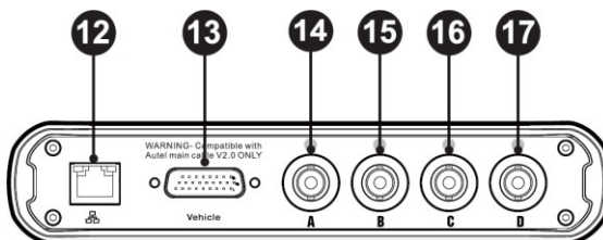
Obrázek 2-6 Spodní pohled na VCM12
