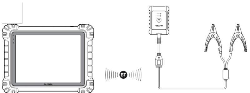
Obrázek 12-3 Příklad připojení testeru baterie 1
