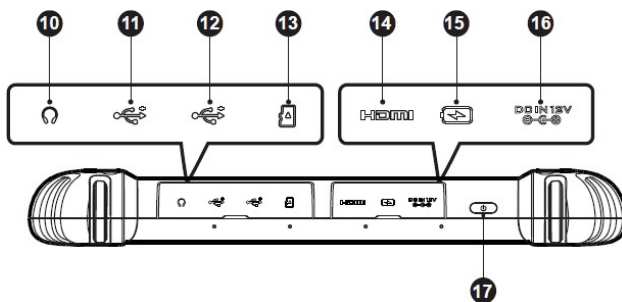
Obrázek 2-3 Tablet MaxiSys, pohled shora
