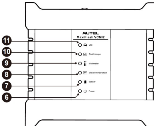
Obrázek 2-5 Přední pohled na VCM12
