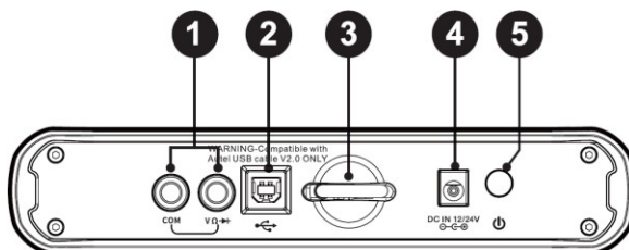
Obrázek 2-4 VCMII2 pohled shora
